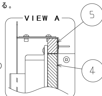
※パッキン挿入位置図（ハッチング部）
