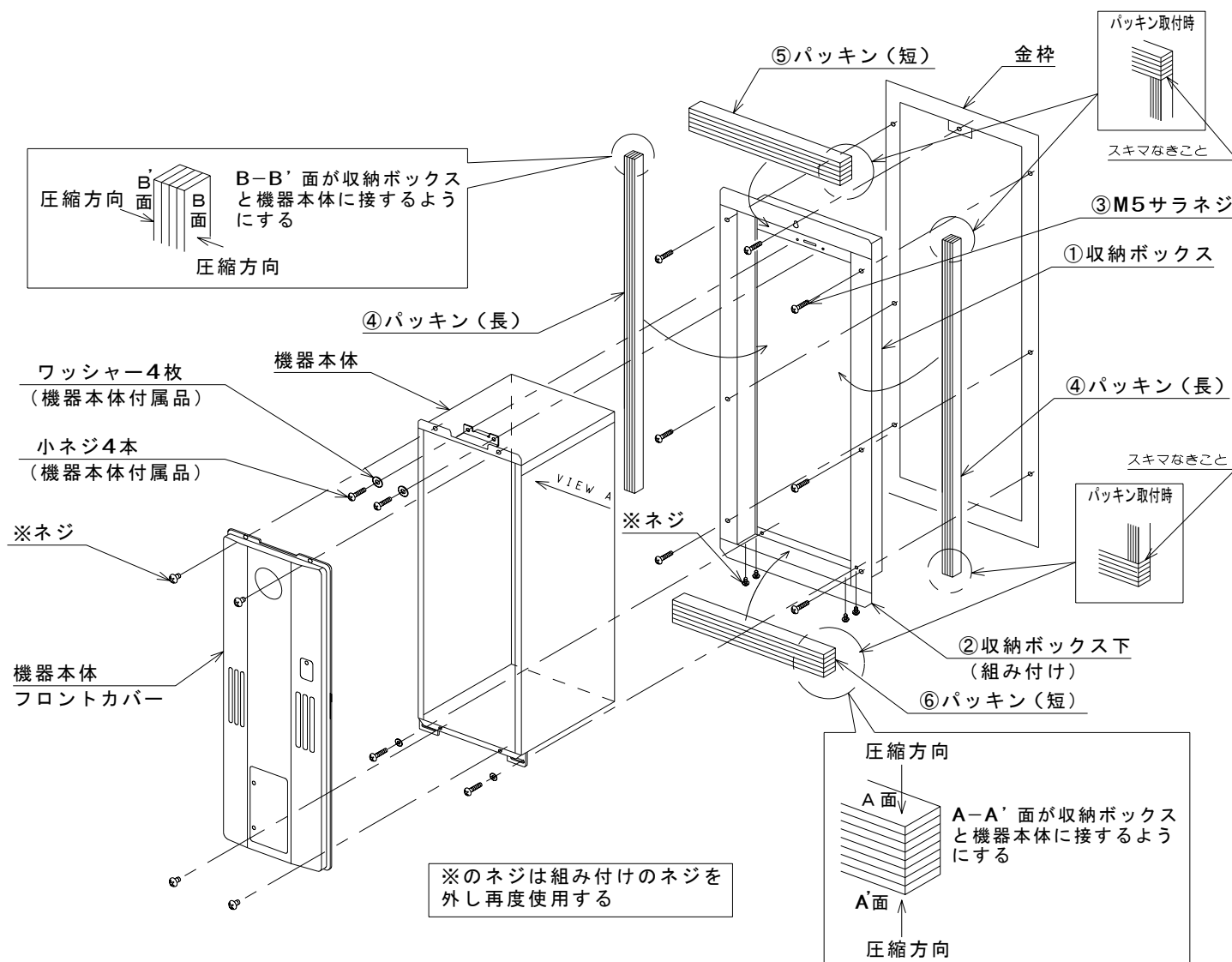
※パッキン挿入位置図（ハッチング部）
