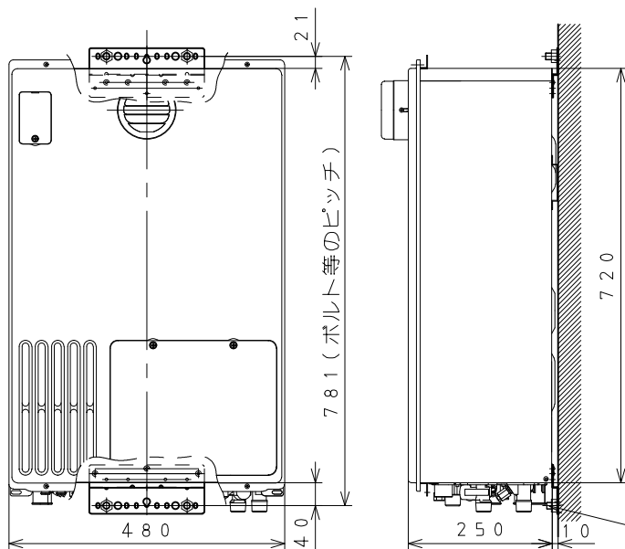
(図3) GH-H240ZWH6 取り付け参考図(単位: mm)
