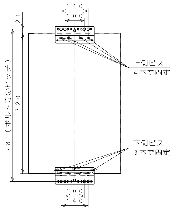
(図2) パーパス製熱源機裏側より(単位: mm)
