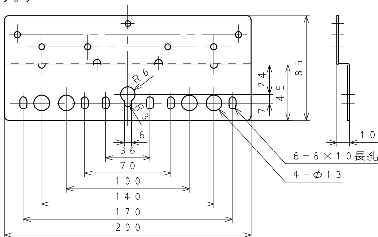
(図1) 取り替え用壁掛け金具(単位: mm)
