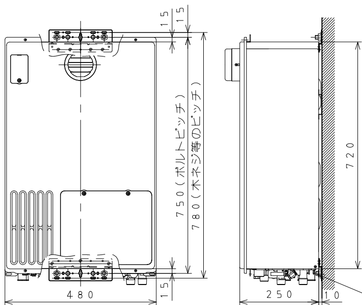
(図3) GH-H240ZW H6 取り付け参考図 (単位：mm)
