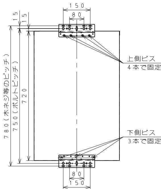
(図2) パーパス製熱源機 裏側より (単位：mm)
