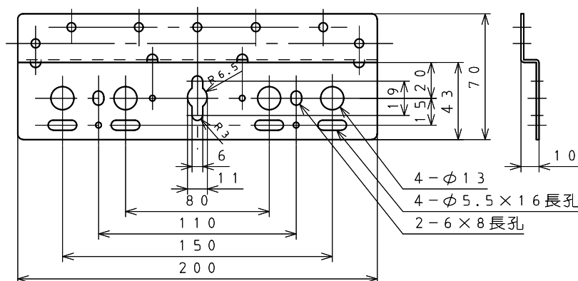
(図1) 取り替え用壁掛け金具 (単位：mm)
