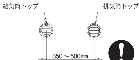
横設置
