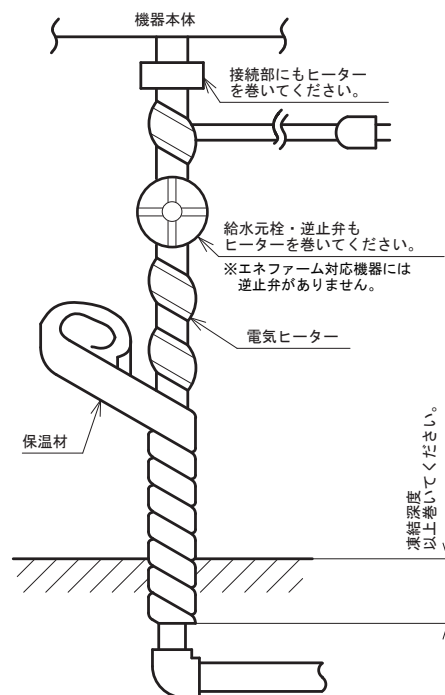
保温材（ヒーター）巻きつけについて
