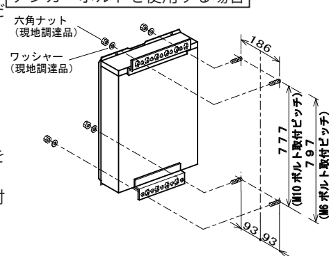
アンカーボルトを使用する場合
