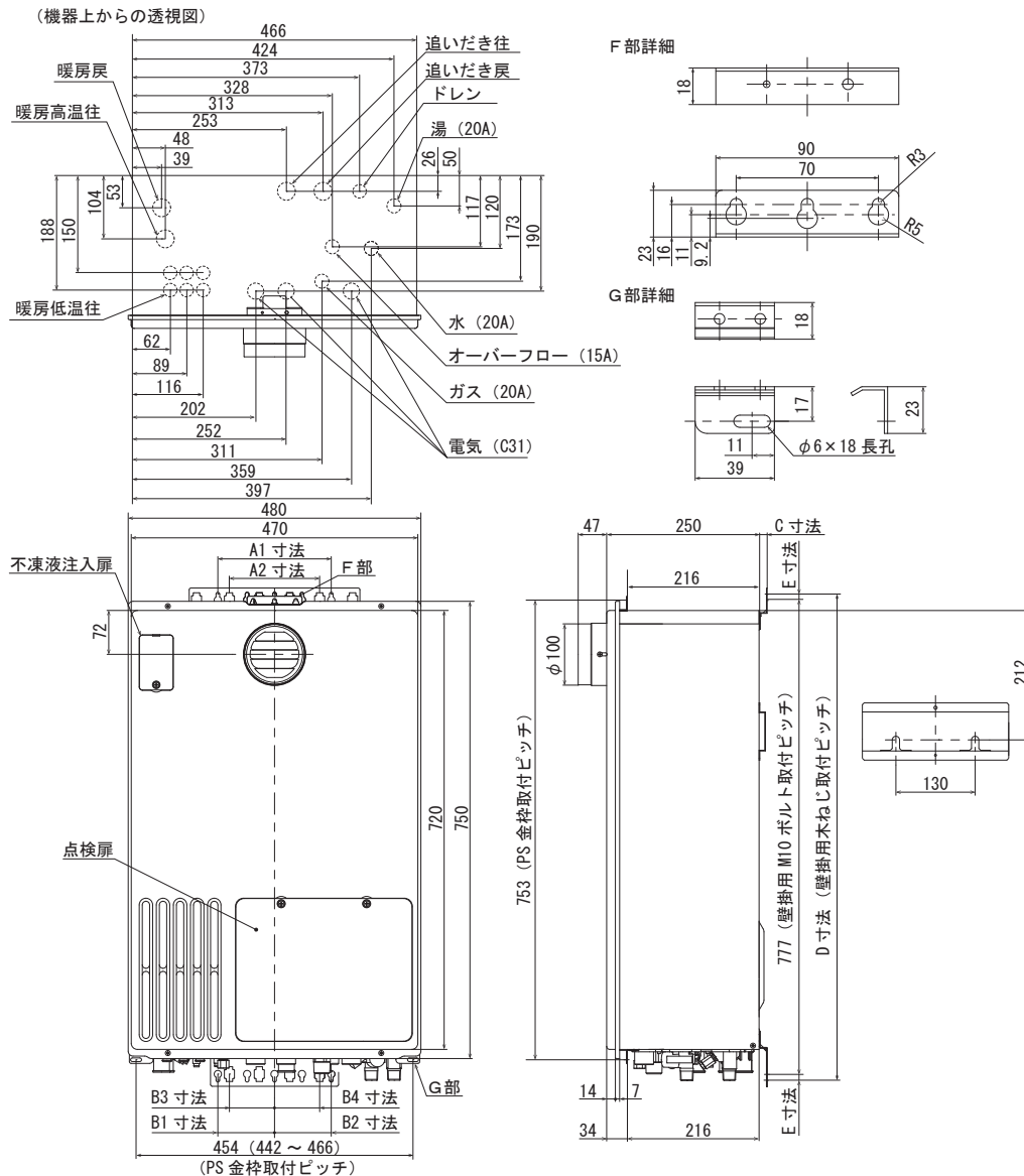
■各配管口径と底板よりの継手高さ (mm)
