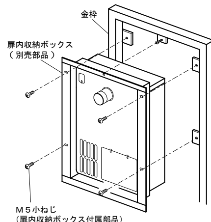
PS 扉内設置の場合
