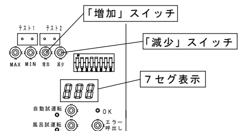
(電装基板)
