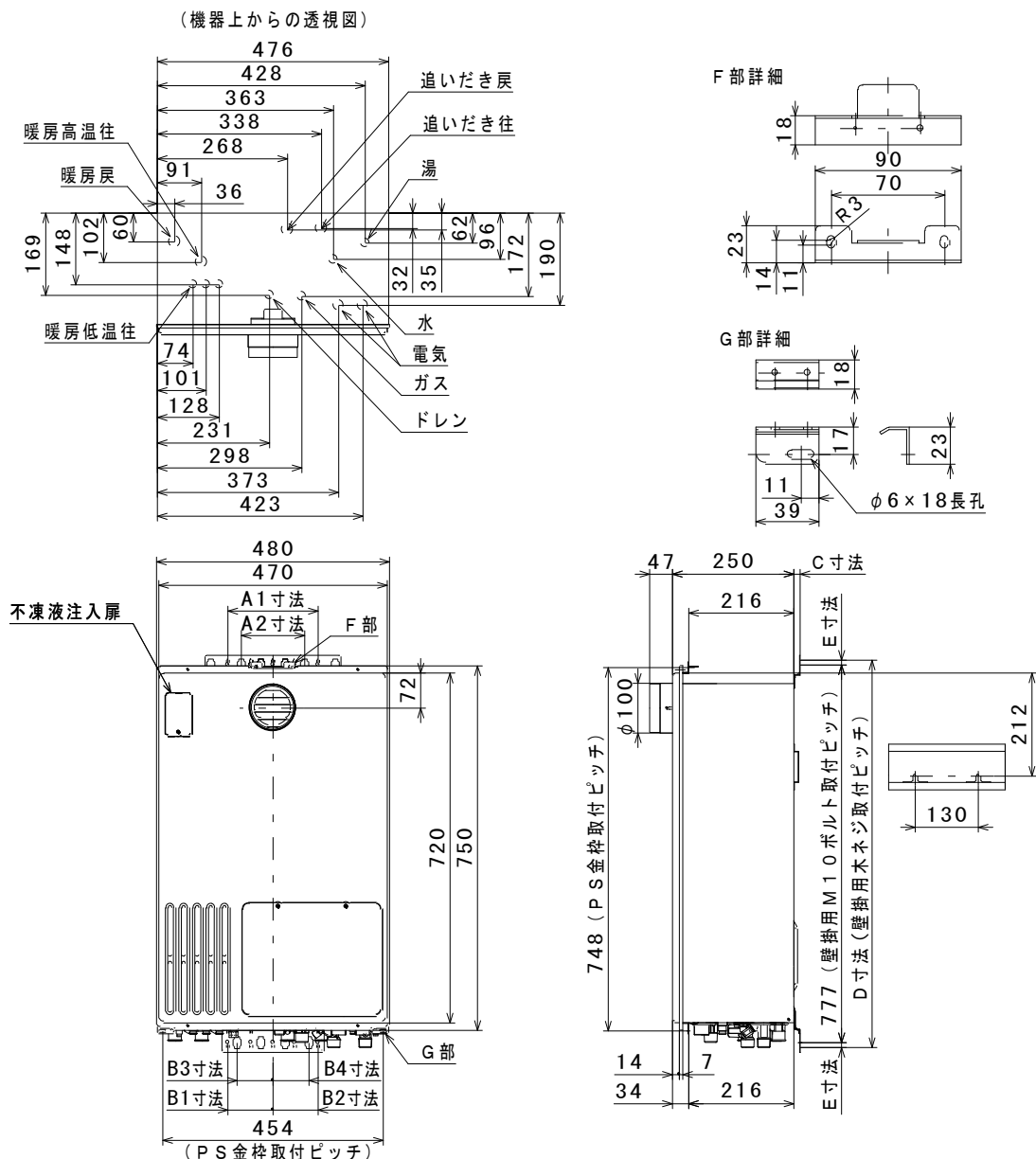
■各配管口径と底板よりの継手高さ(mm)
