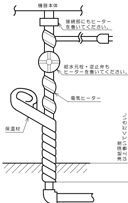
保温材(ヒーター)巻きつけについて
