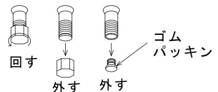
水抜き栓 (6) の外し方
