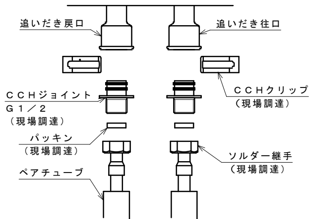
銅管接続の場合
