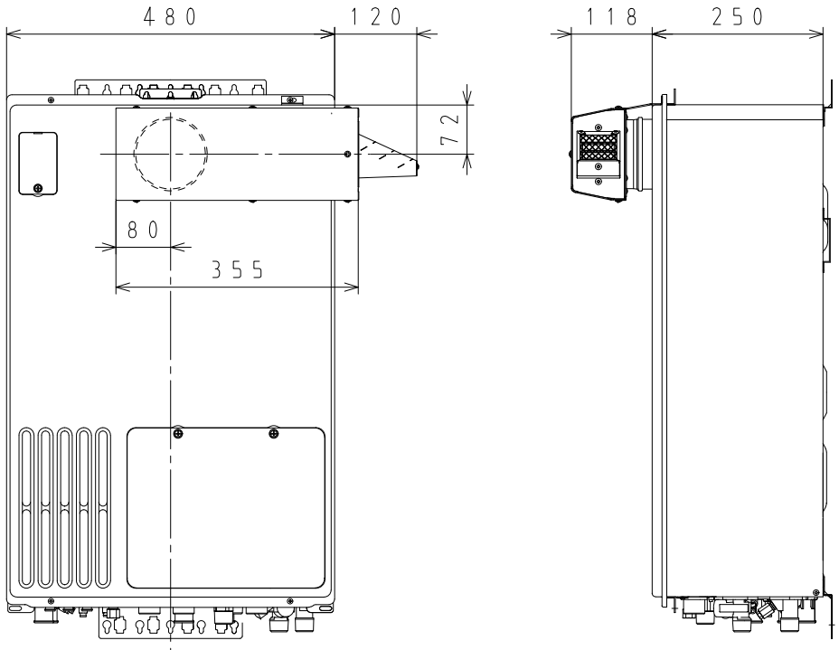
③ ( G H - H 2 4 0 Z Y ) + ( Y A - U 3 0 ) 取付寸法図 ( 単位 : mm )
