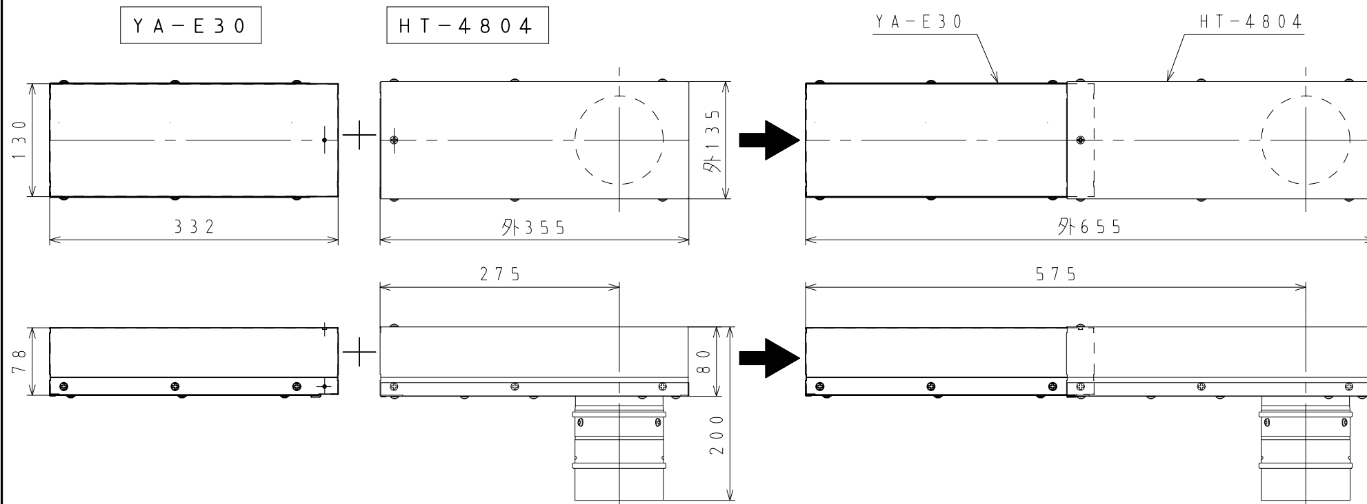
② ( H T - 4 8 0 4 ) + ( Y A - E 3 0 ) 取付寸法図 ( 単位 : mm )
