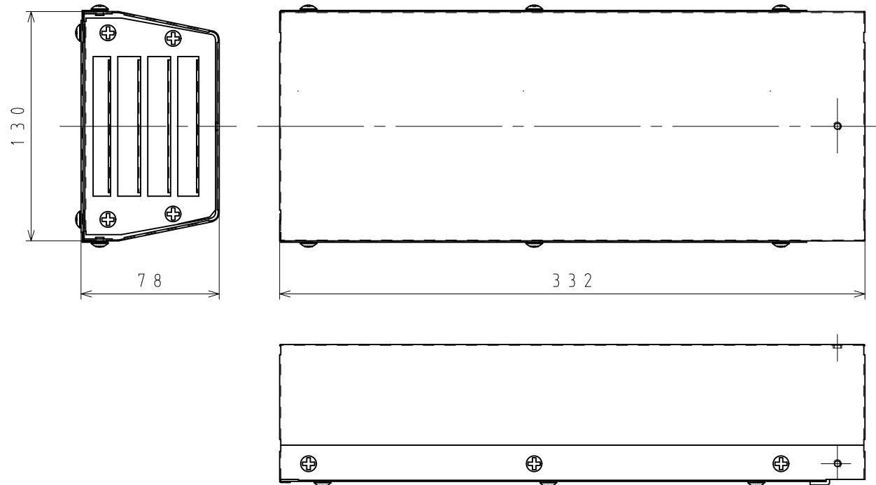
① Y A - E 3 0 本体寸法図 ( 単位 : mm )
