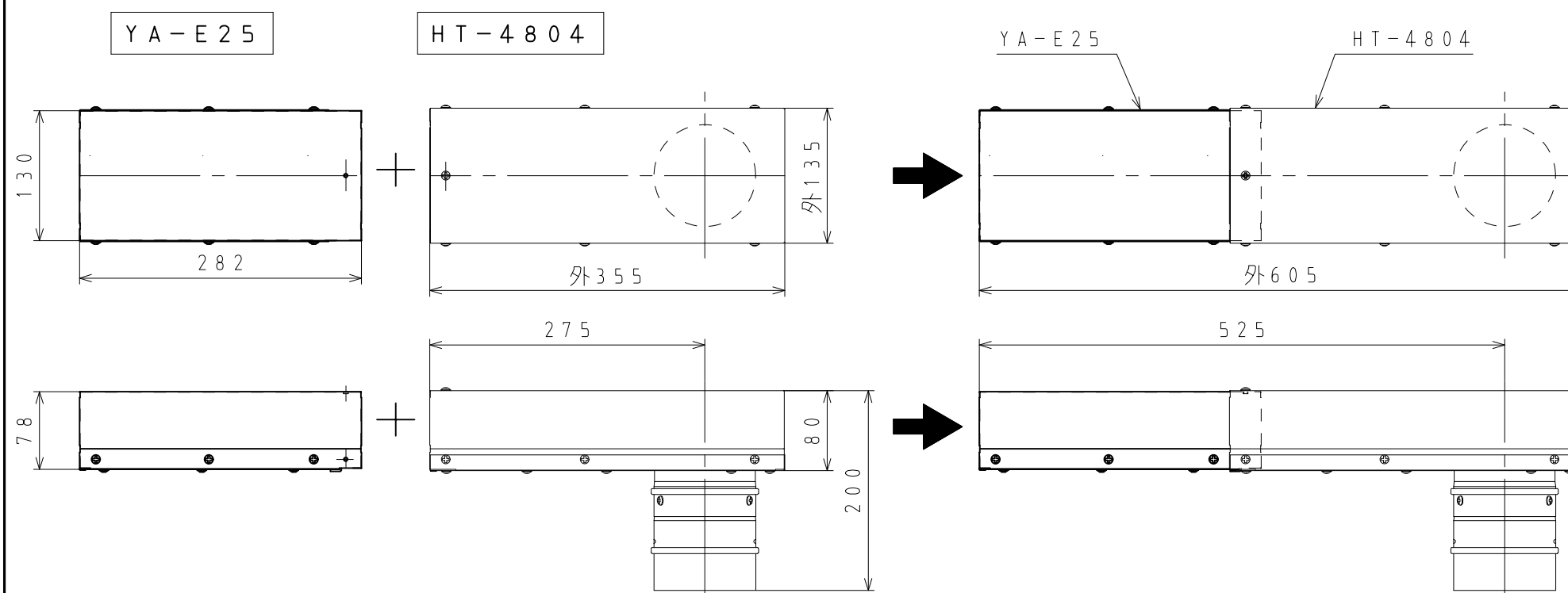
② ( H T - 4 8 0 4 ) + ( Y A - E 2 5 ) 取付寸法図 ( 単位 : mm )
