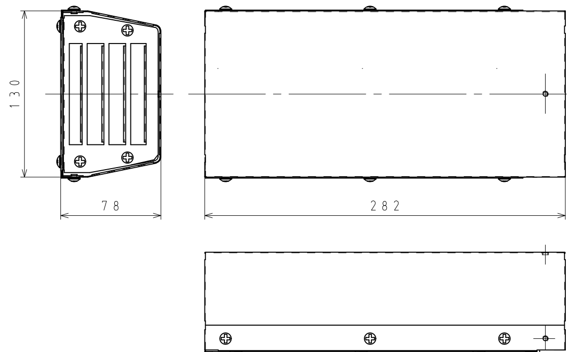
① Y A - E 2 5 本体寸法図 ( 単位 : mm )
