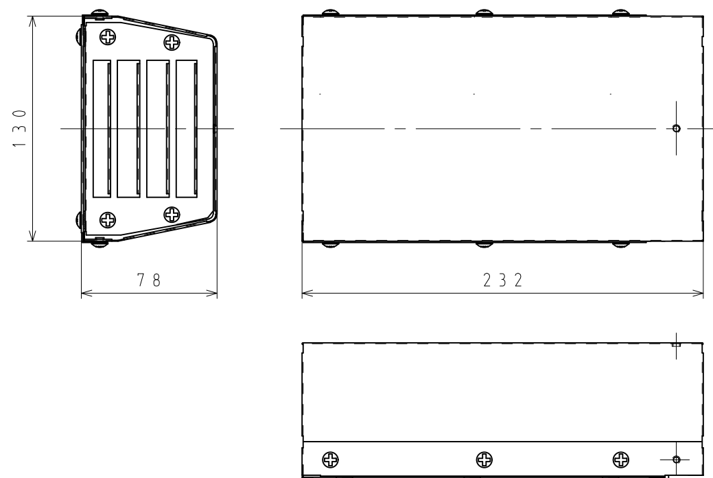
① Y A - E 2 0 本体寸法図 ( 単位 : mm )
