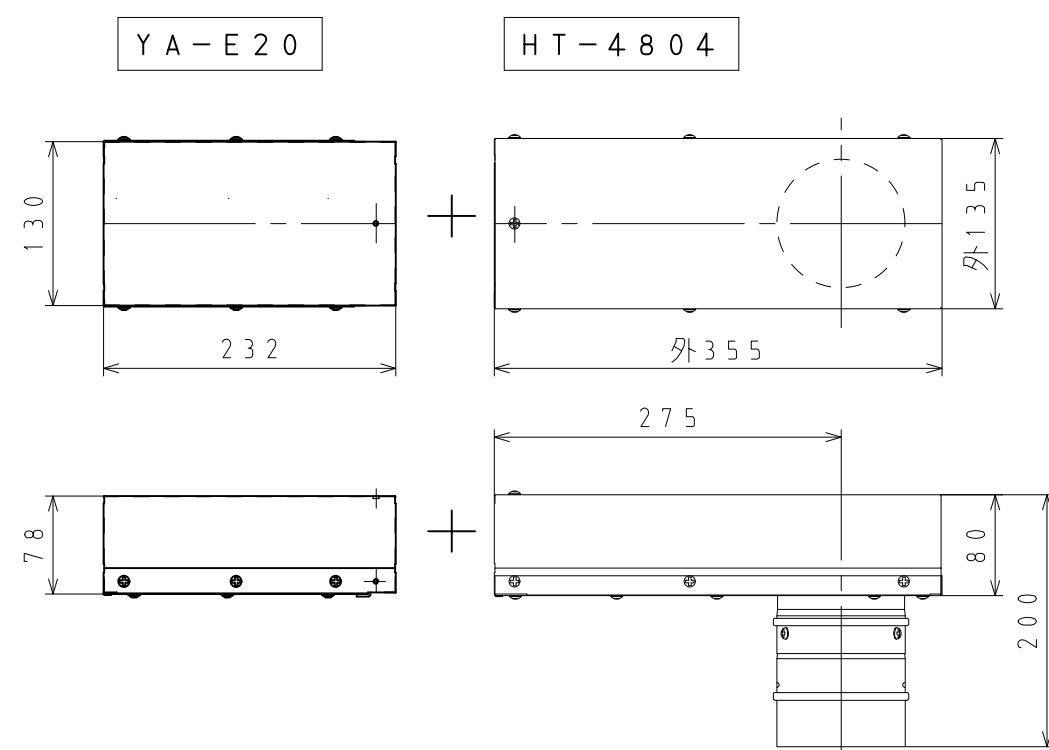
② ( H T - 4 8 0 4 ) + ( Y A - E 2 0 ) 取付寸法図 ( 単位 : mm )
