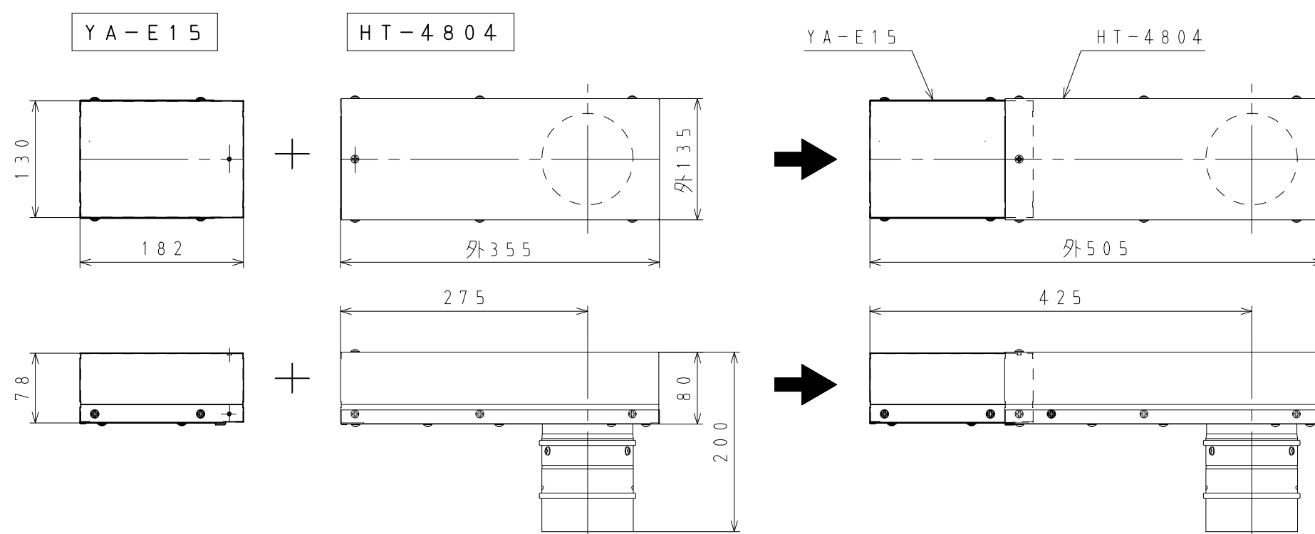
② ( H T - 4 8 0 4 ) + ( Y A - E 1 5 ) 取付寸法図 ( 単位 : mm )
