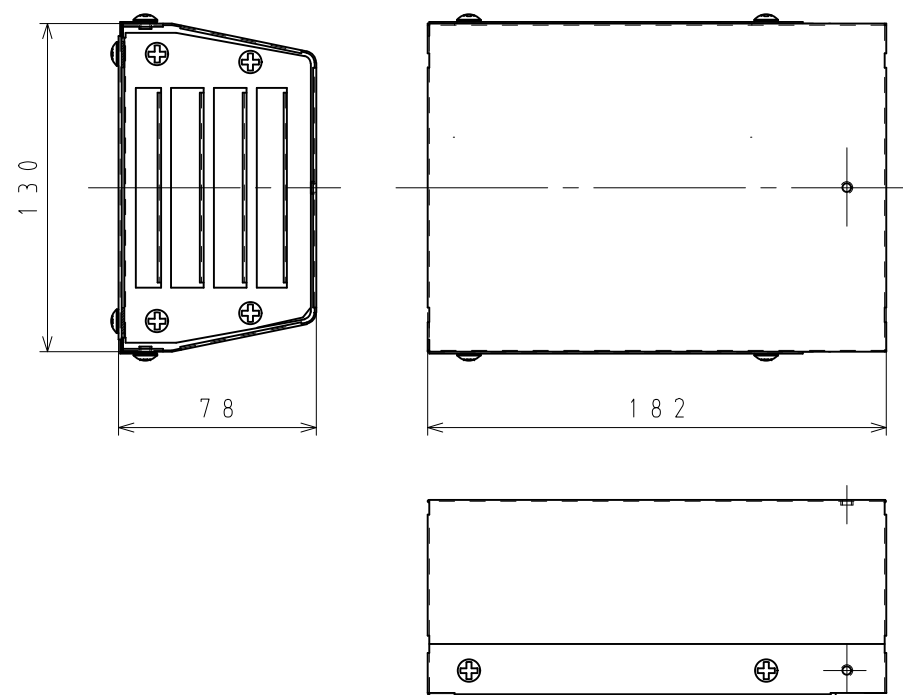
① Y A - E 1 5 本体寸法図 ( 単位 : mm )
