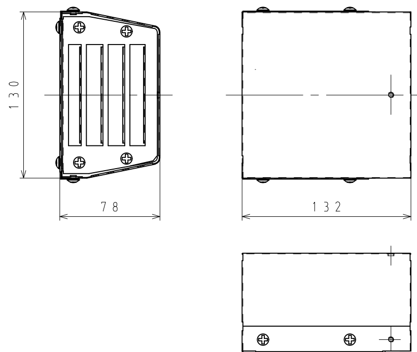
① Y A - E 1 0 本体寸法図 ( 単位 : mm )
