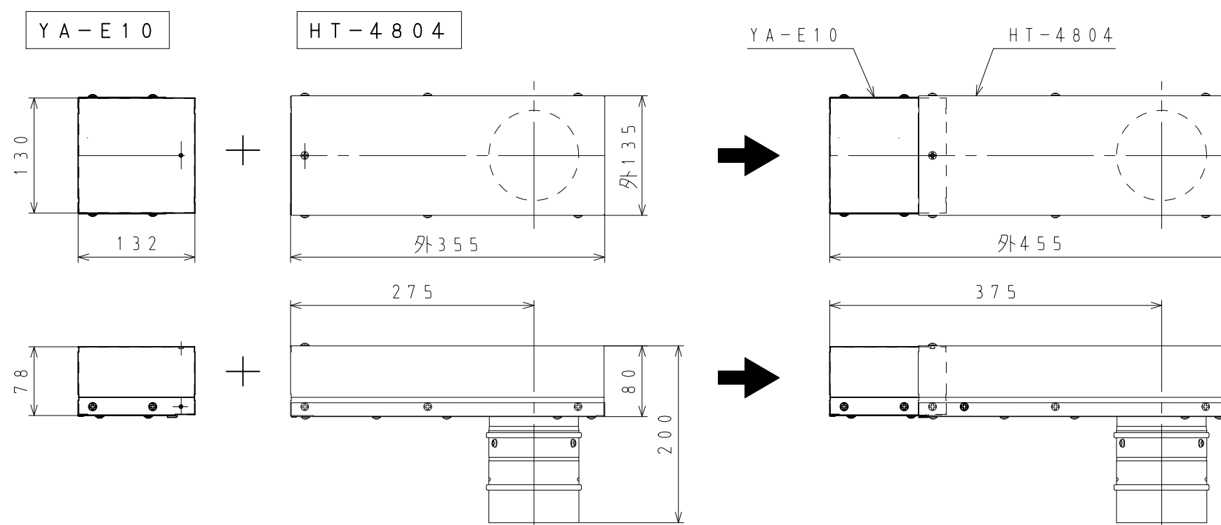
② ( H T - 4 8 0 4 ) + ( Y A - E 1 0 ) 取付寸法図 ( 単位 : mm )
