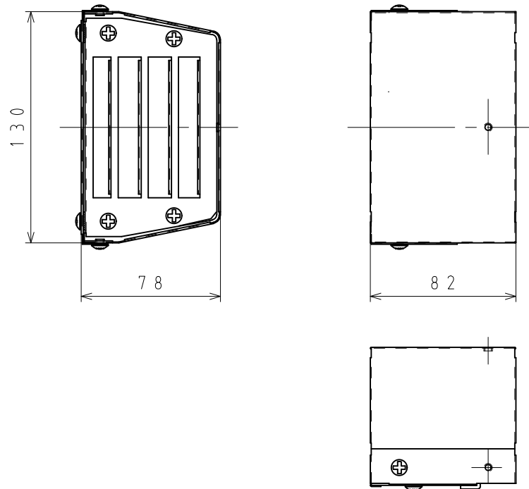
① Y A - E 0 5 本体寸法図 ( 単位 : mm )
