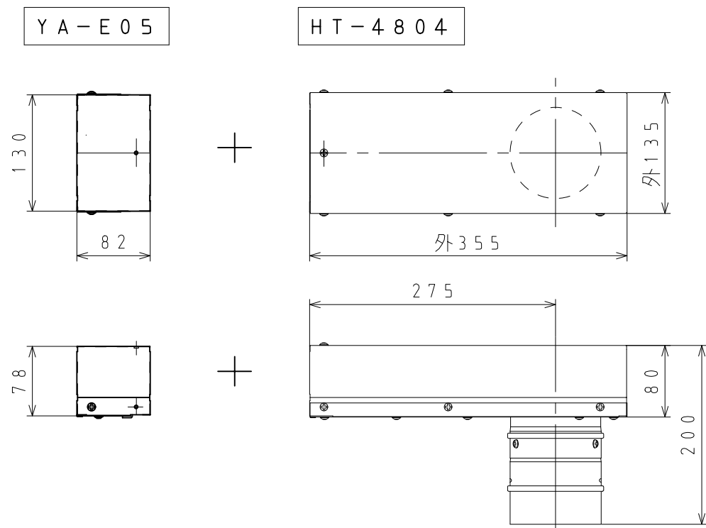
② ( H T - 4 8 0 4 ) + ( Y A - E 0 5 ) 取付寸法図 ( 単位 : mm )
