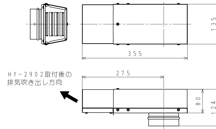
③HT-4803 取付寸法図（単位：mm）
