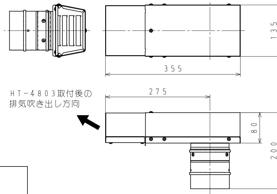
③HT-4803 取付寸法図（単位：mm）
