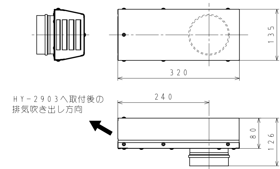
③HT-4804 取付寸法図（単位：mm）
