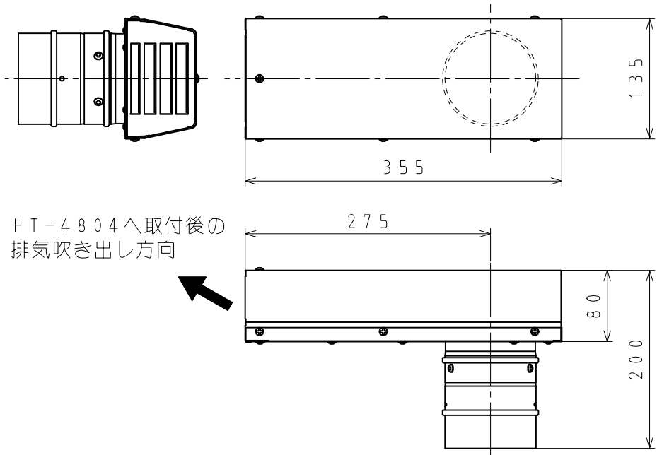
③HT-4804 取付寸法図（単位：mm）
