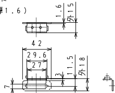
①A部詳細(板厚1.6)
