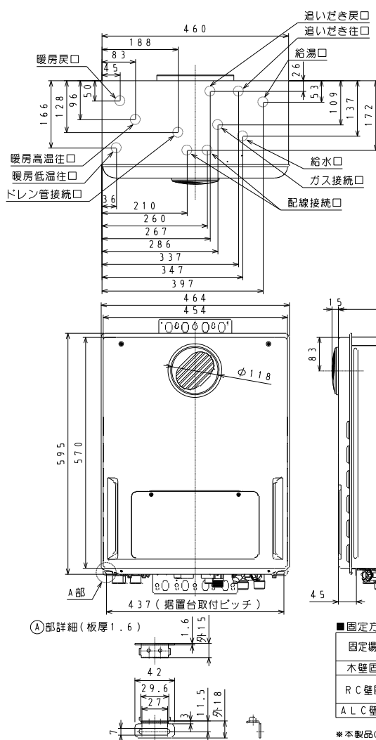
■底板よりの各継手高さ・各配管口径
