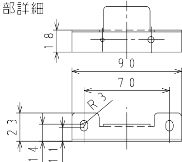
G 部詳細
