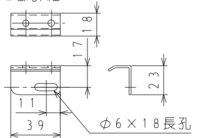
H 部詳細
