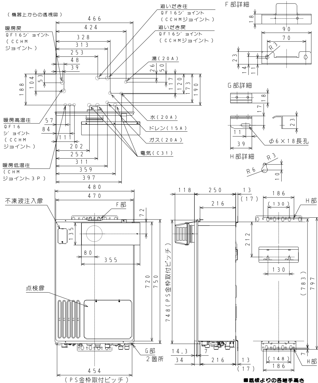
■底板よりの各継手高さ (mm)
