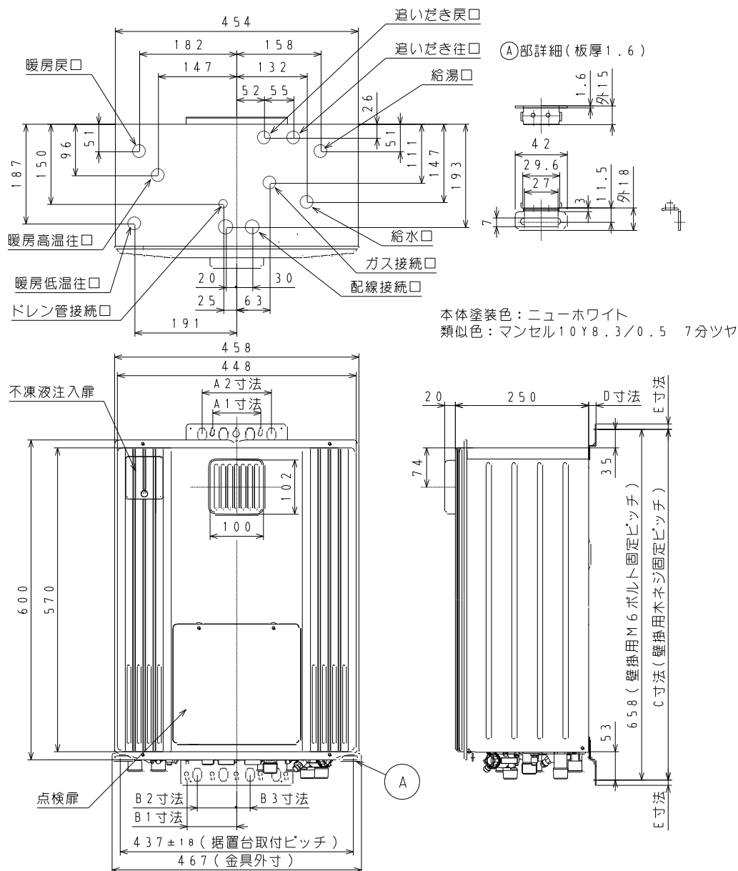
■底板よりの各継手高さ・各配管口径
