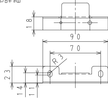
G 部詳細
