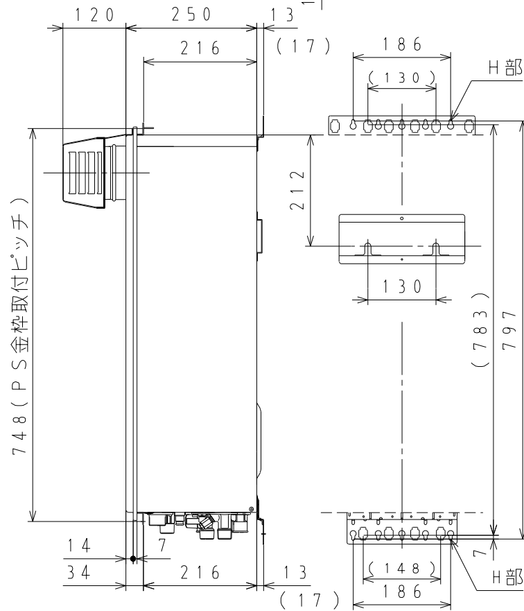
■固定方法と部材仕様
