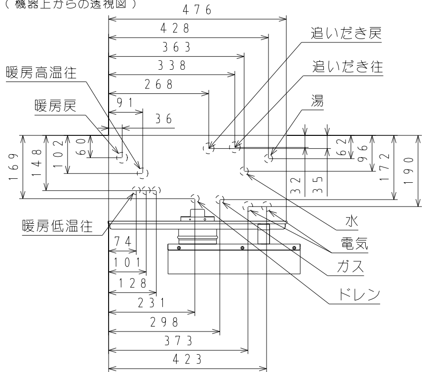
■機器本体寸法図（単位：mm）本図は排気右吹き出しの場合を示す（機器上からの透視図）
