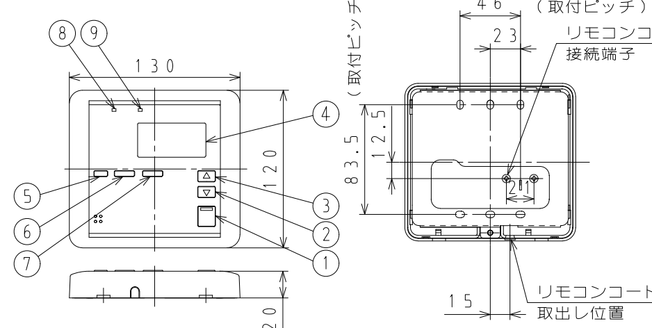
② 温水温度リモコン寸法図（別売部品） （FHR-18）
