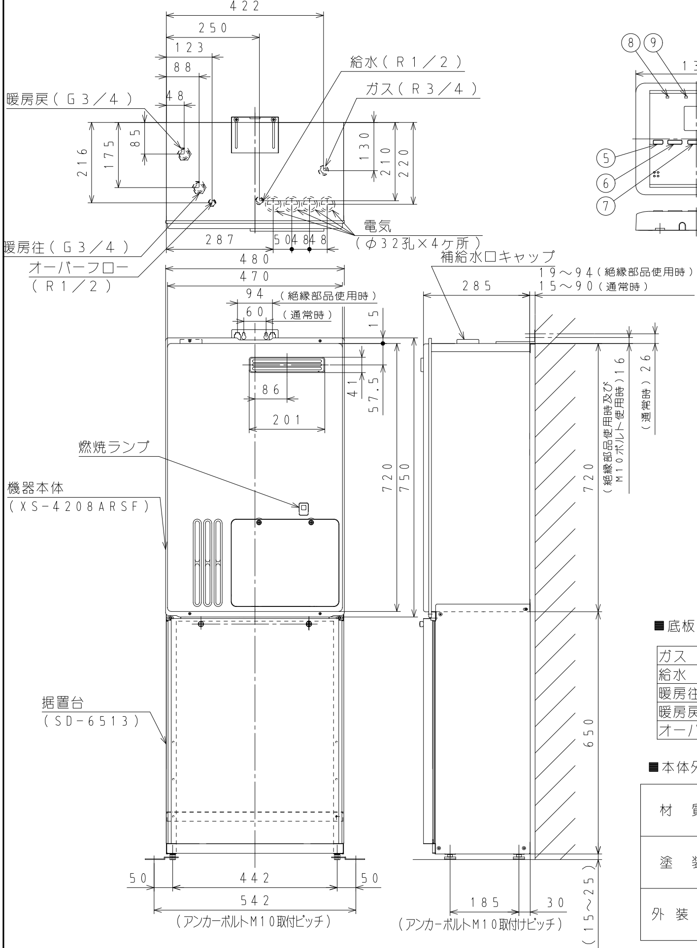
① 機器本体寸法図（単位：mm）
