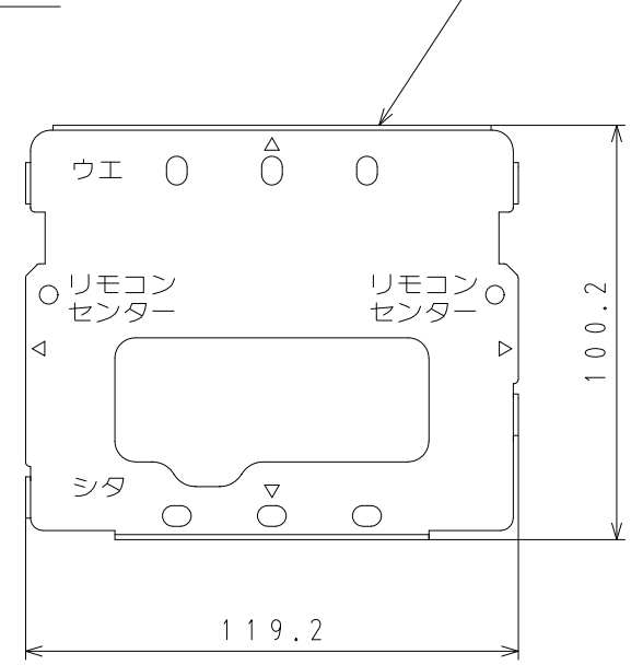
壁取付金具 寸法図
