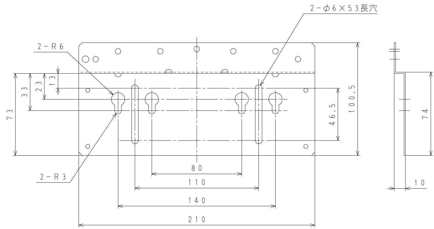
①-1 本体寸法図 (単位: mm)
