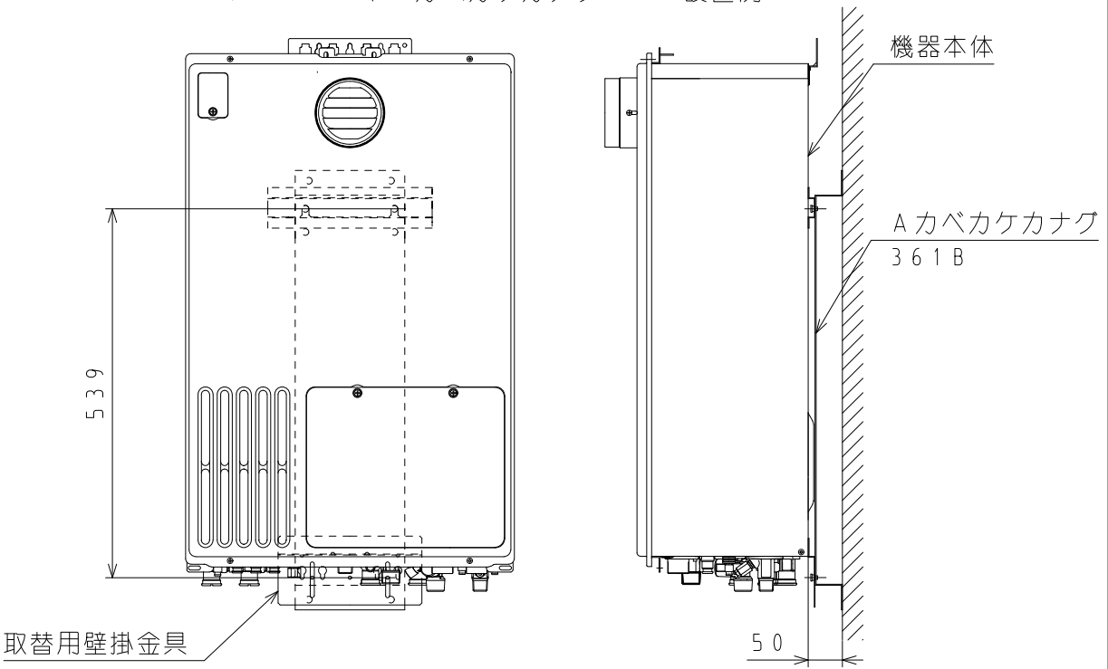
①-2 製品取付参考図
