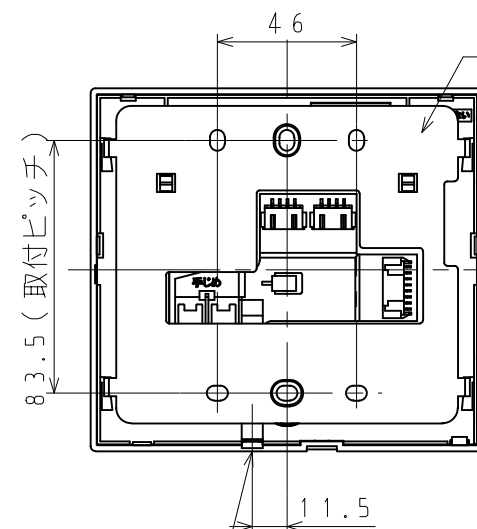
壁取付金具
