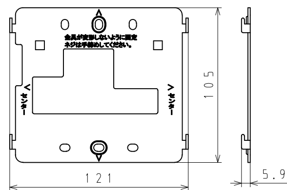
壁取付金具 寸法図
