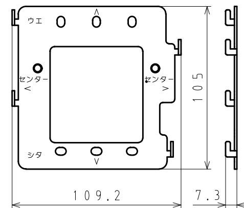
壁取付金具 寸法図
