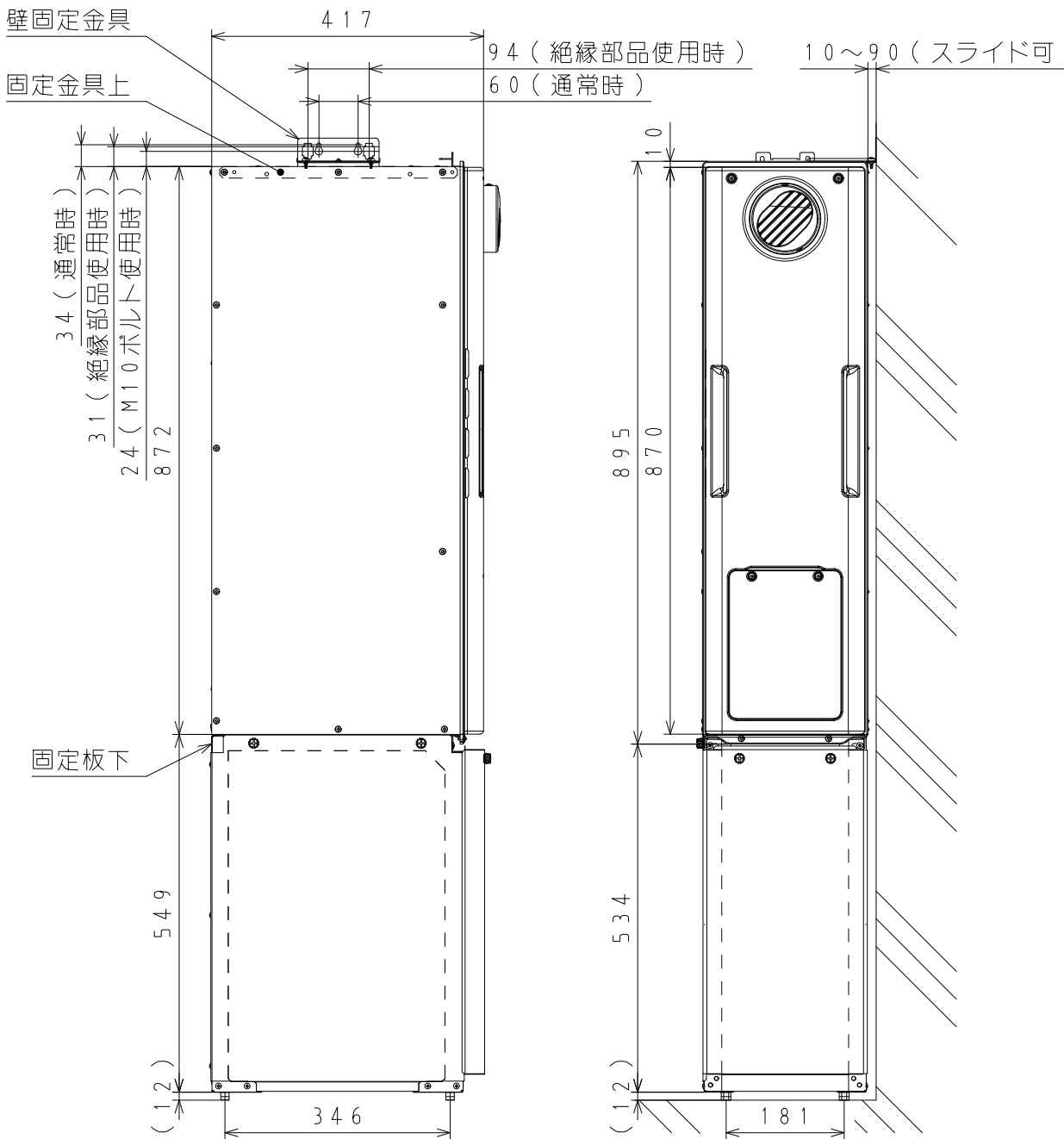
②取付寸法図
