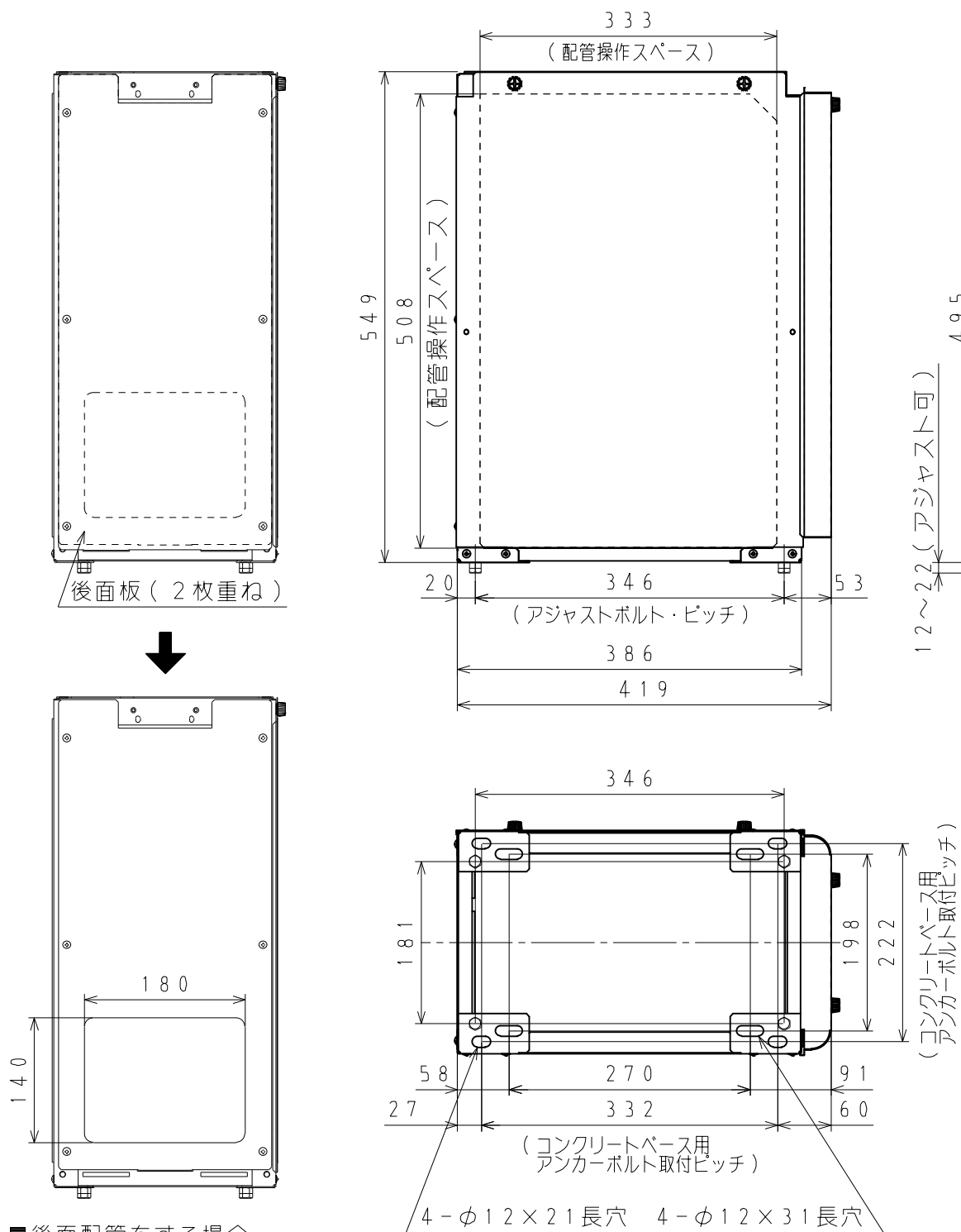
■固定方法と部材仕様
