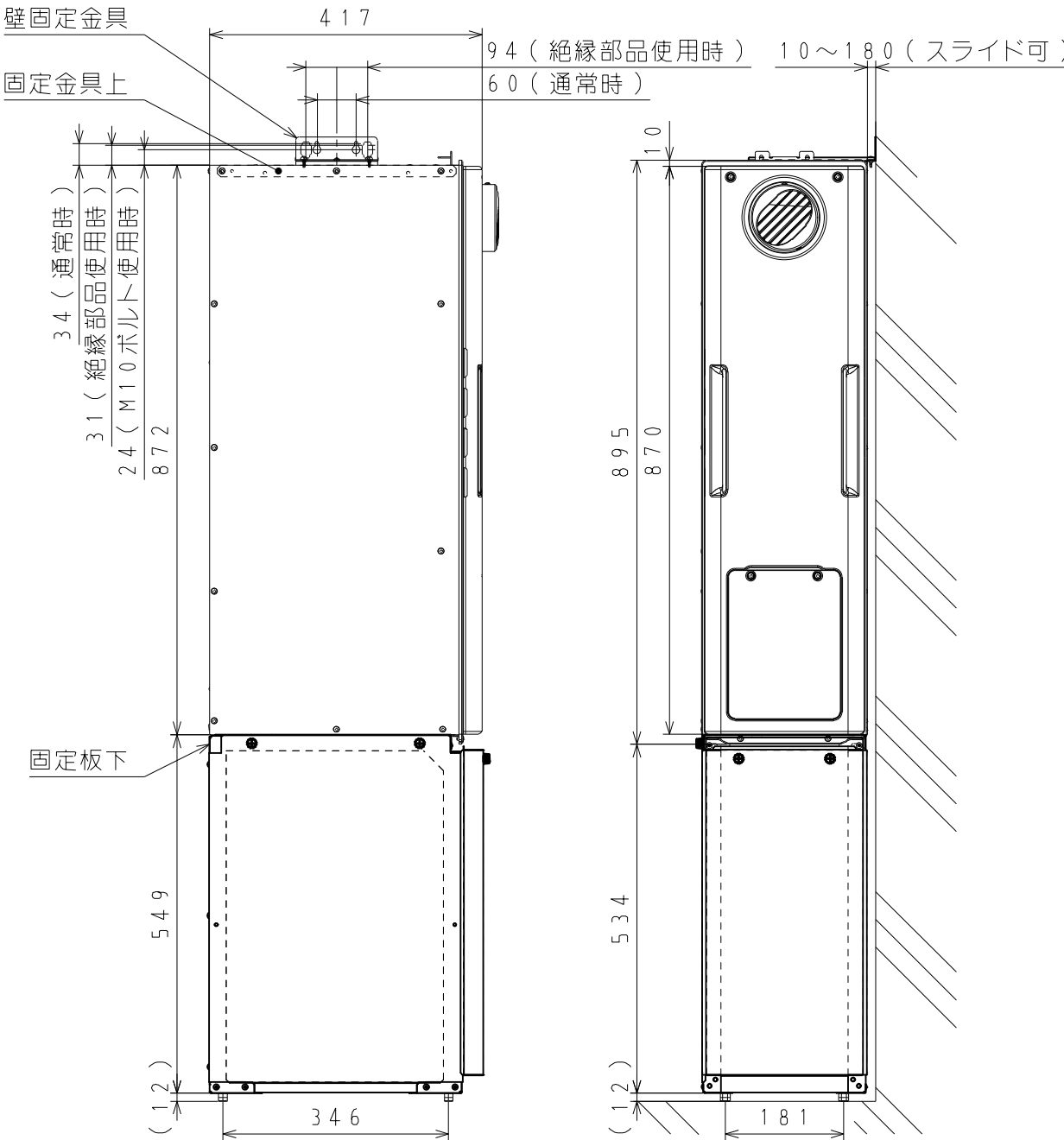
②取付寸法図 XT4220LRS AW4C取付設置例
