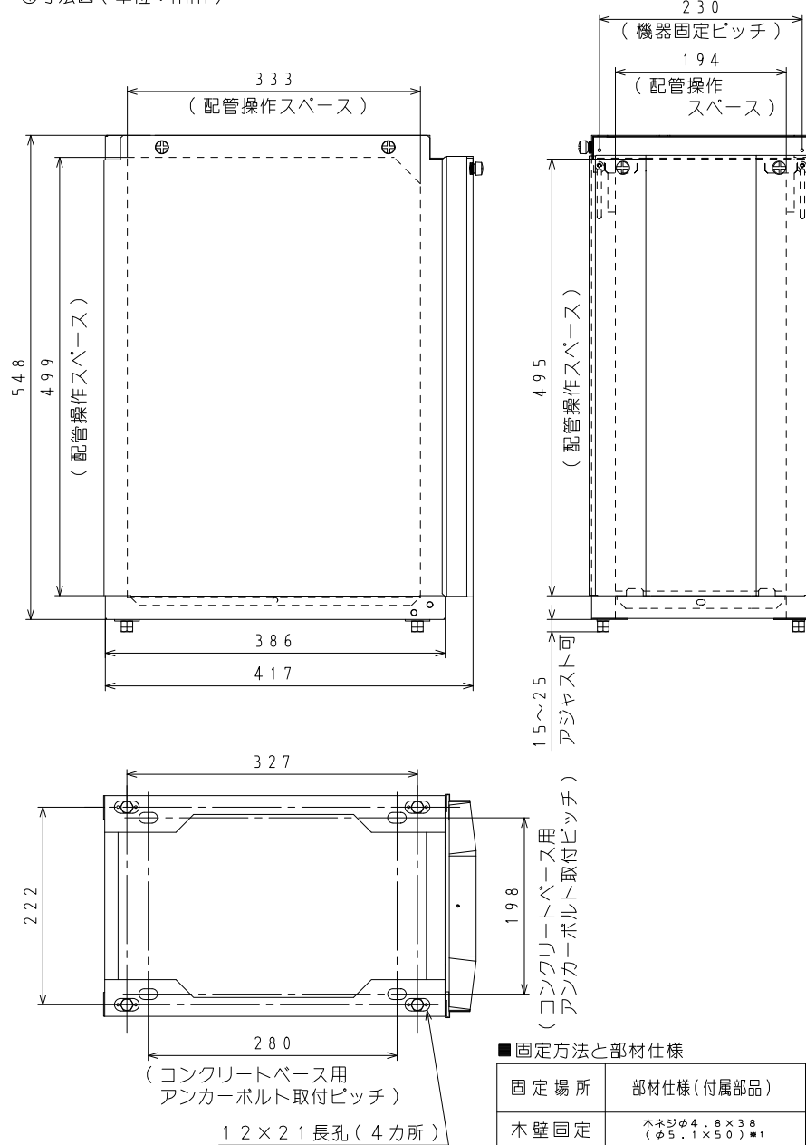
①寸法図 (単位: mm)
