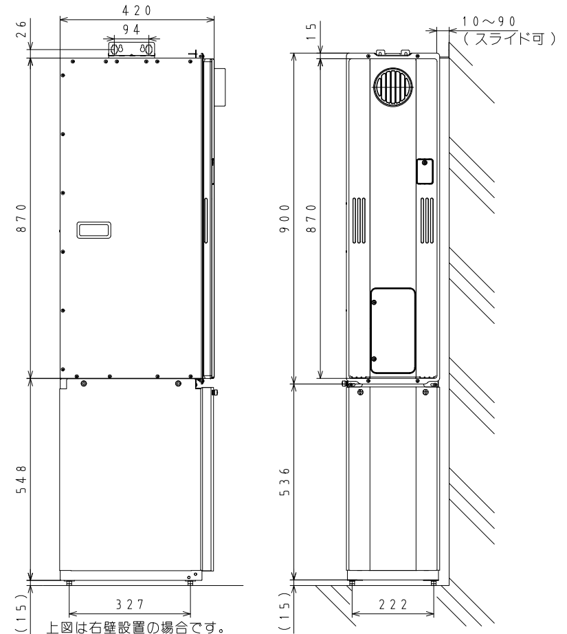
②取付寸法図 (GH-H2400ZWS取付例)
