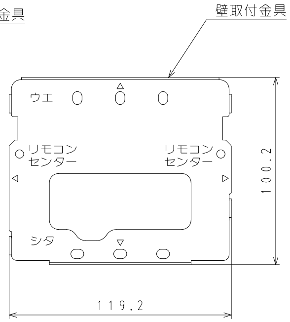
壁取付金具 寸法図
