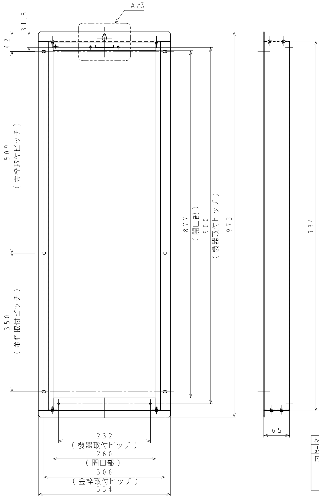
① 本体寸法図 (単位: mm)
