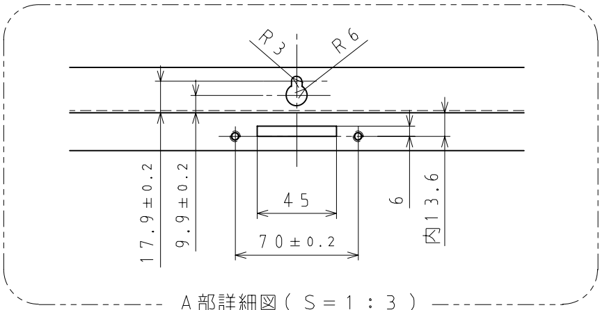
② 機器取付参考図
