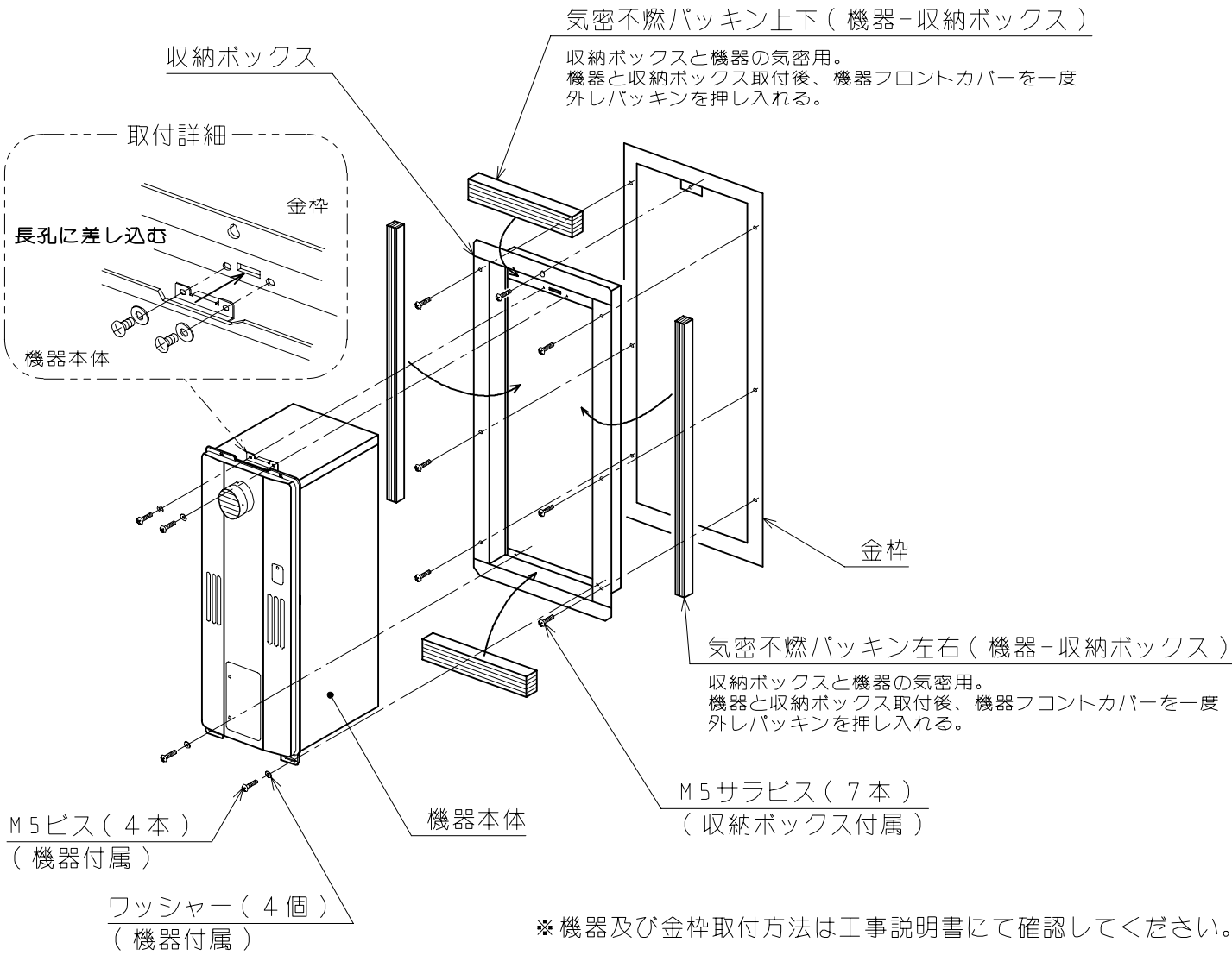
② 機器取付参考図
