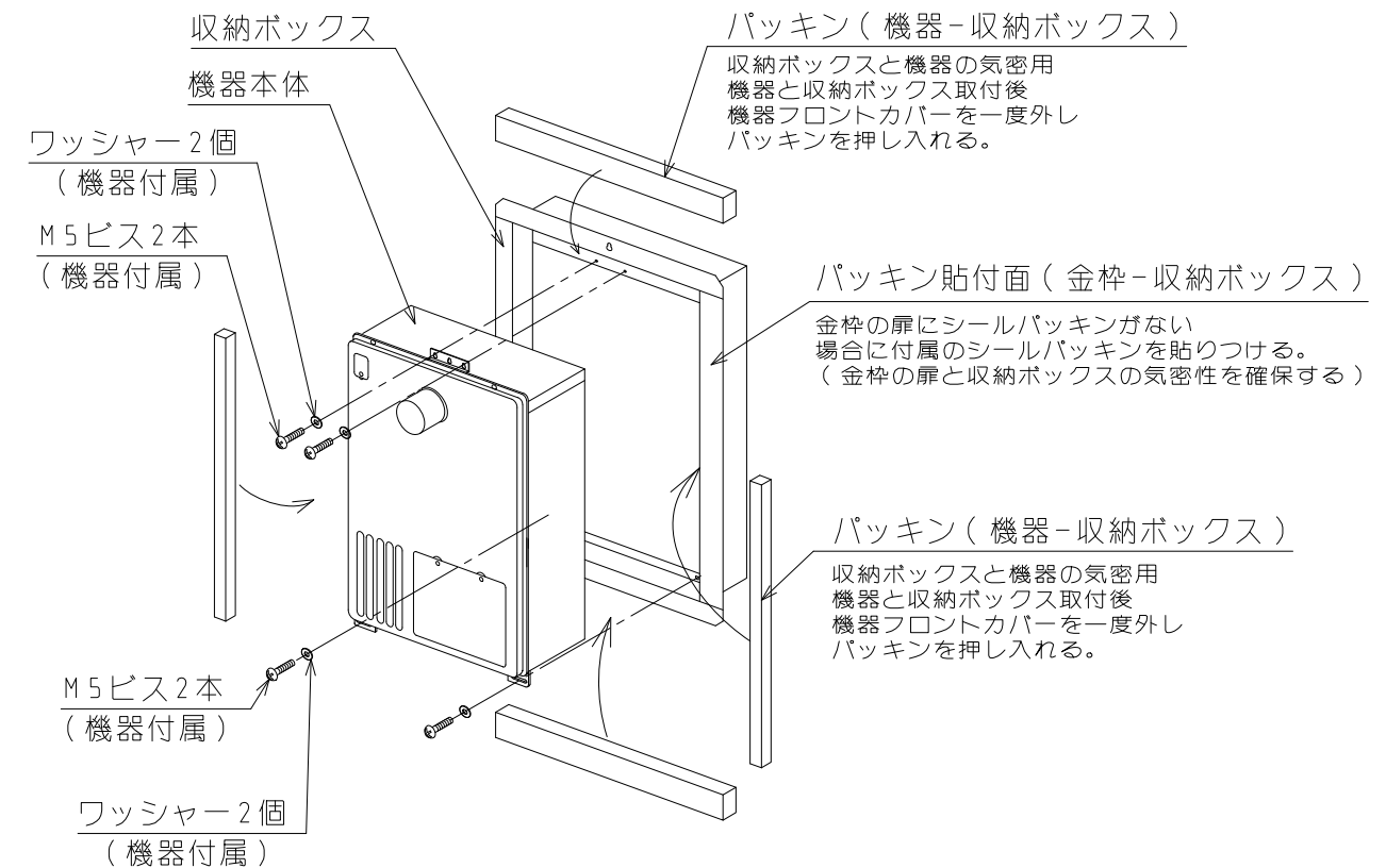
①-2 製品取付参考図
