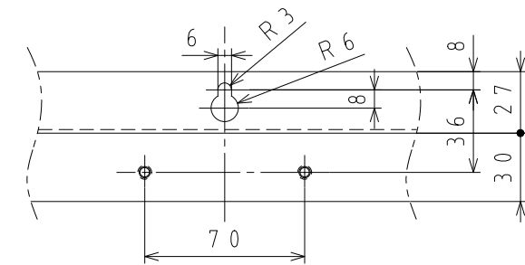
A部詳細図 (単位: mm)
