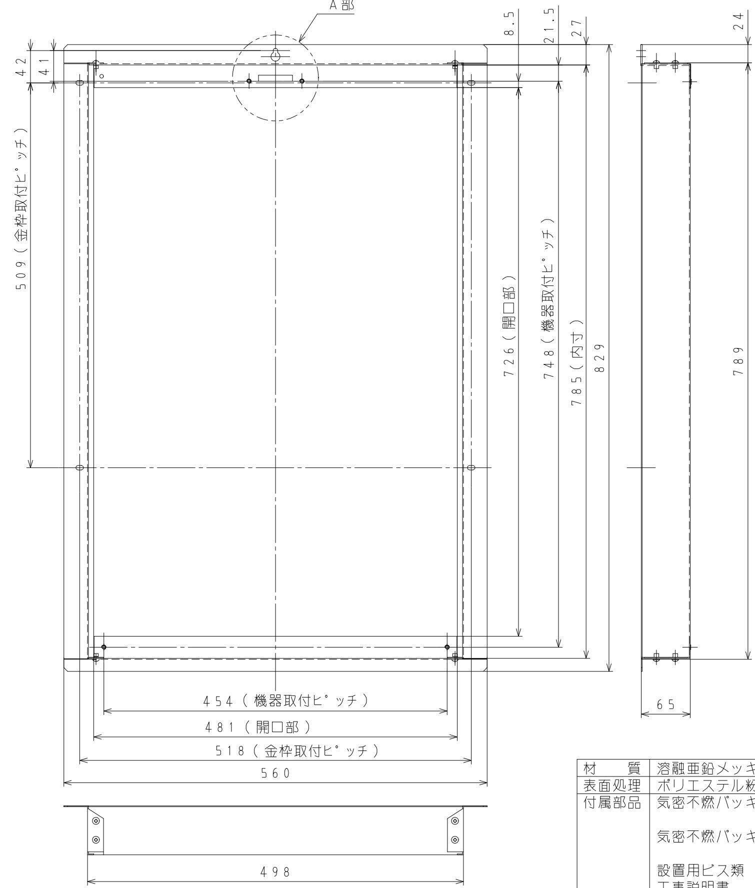
①-1 本体寸法図 (単位: mm)
