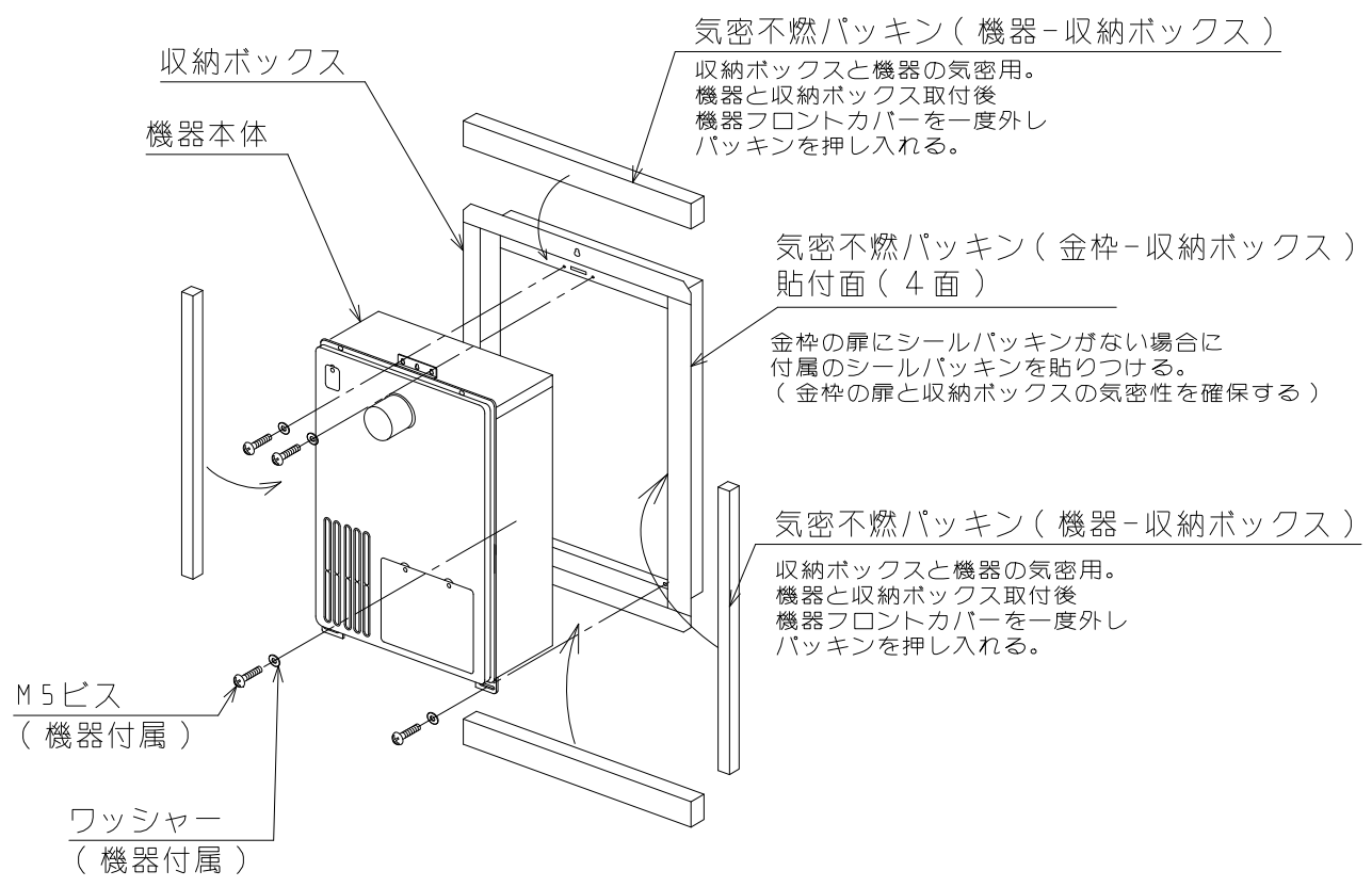
①-2 機器取付参考図
