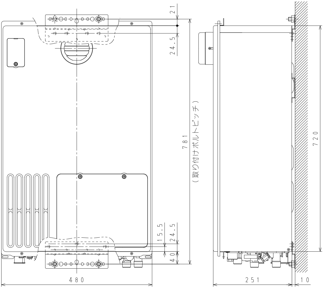
①-2 GH-H240ZWH6 取り付け参考図 (S=1:6 単位:mm)
