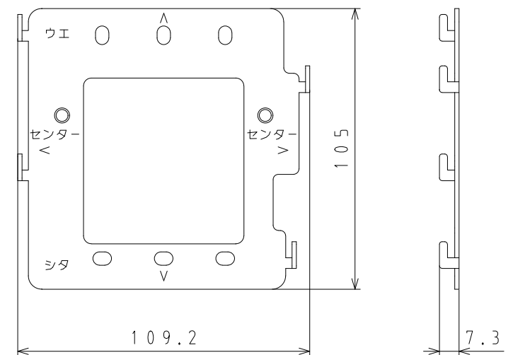
壁取付金具 寸法図
