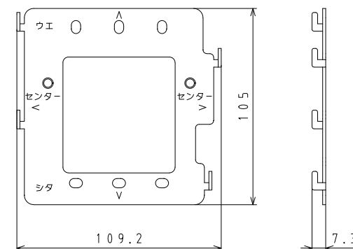
材質：LGD 板厚： t=1.6
