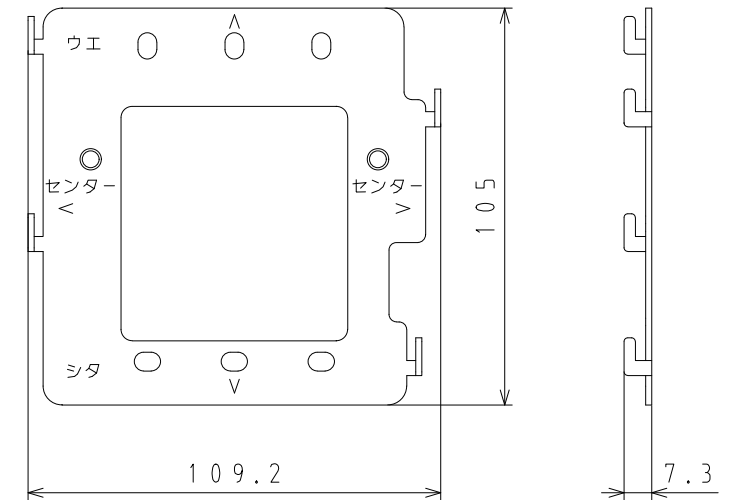
壁取付金具 寸法図
