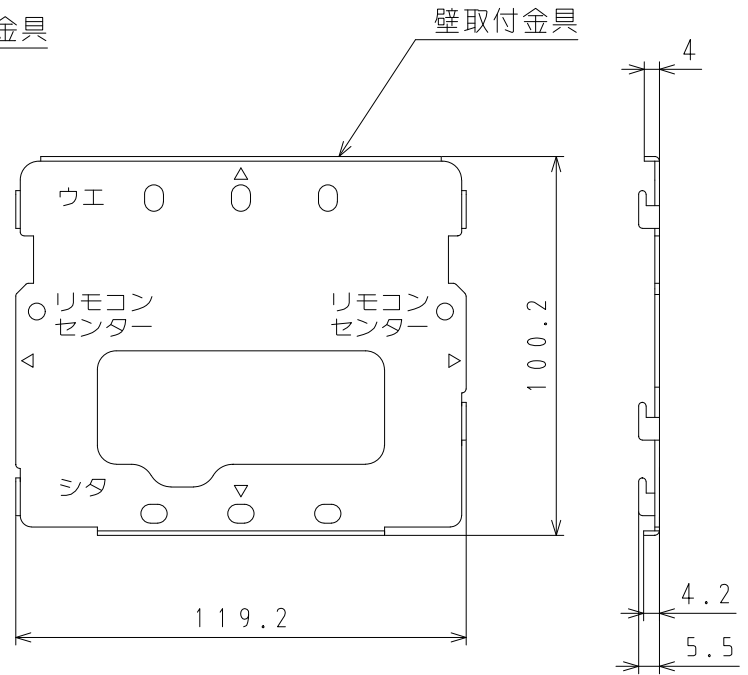
壁取付金具 寸法図 材質: LGD 板厚: t1.2
