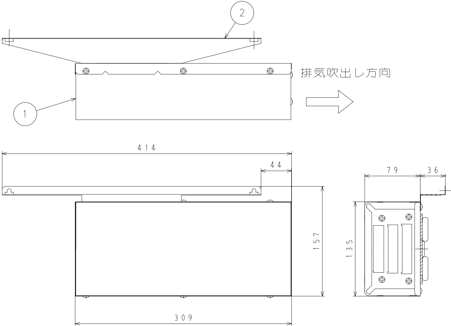
1 本体寸法図(単位:mm)
