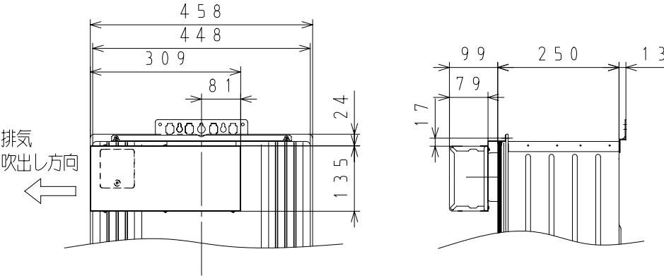
2-2 GH-HK2400ZW GH-HK2400AW 取付寸法図 (排气左出しの場合)
