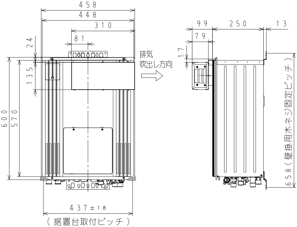
2-1 GH-HK2400ZW GH-HK2400AW 取付寸法図 (排气右出しの場合)
