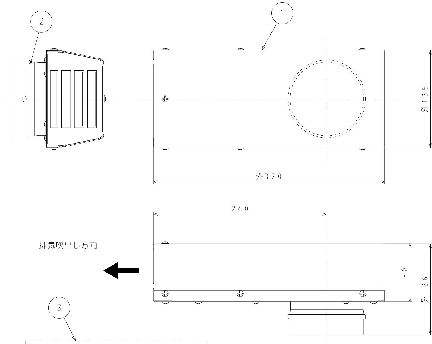
①本体寸法図（単位：mm）
