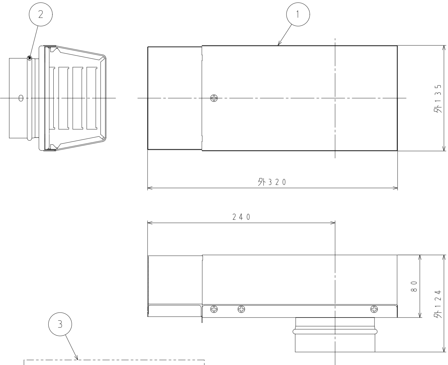
①本体寸法図(単位:mm)
