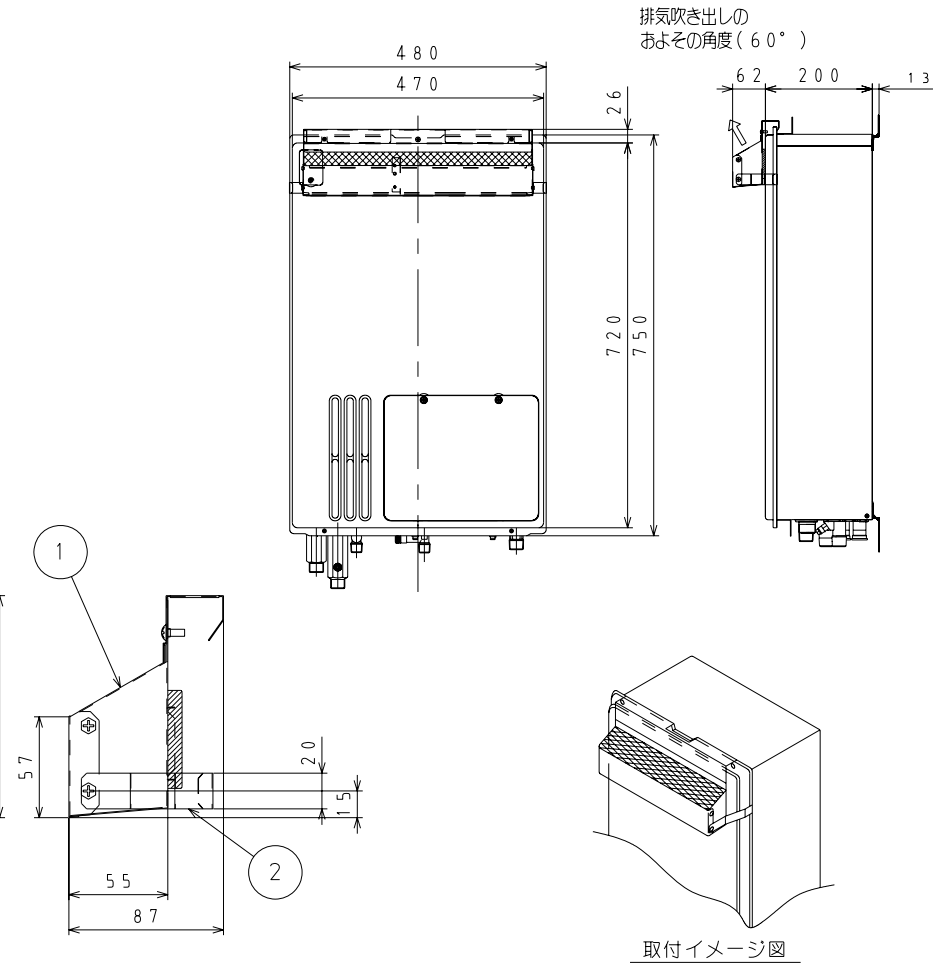
② 取付け例：寸法図
