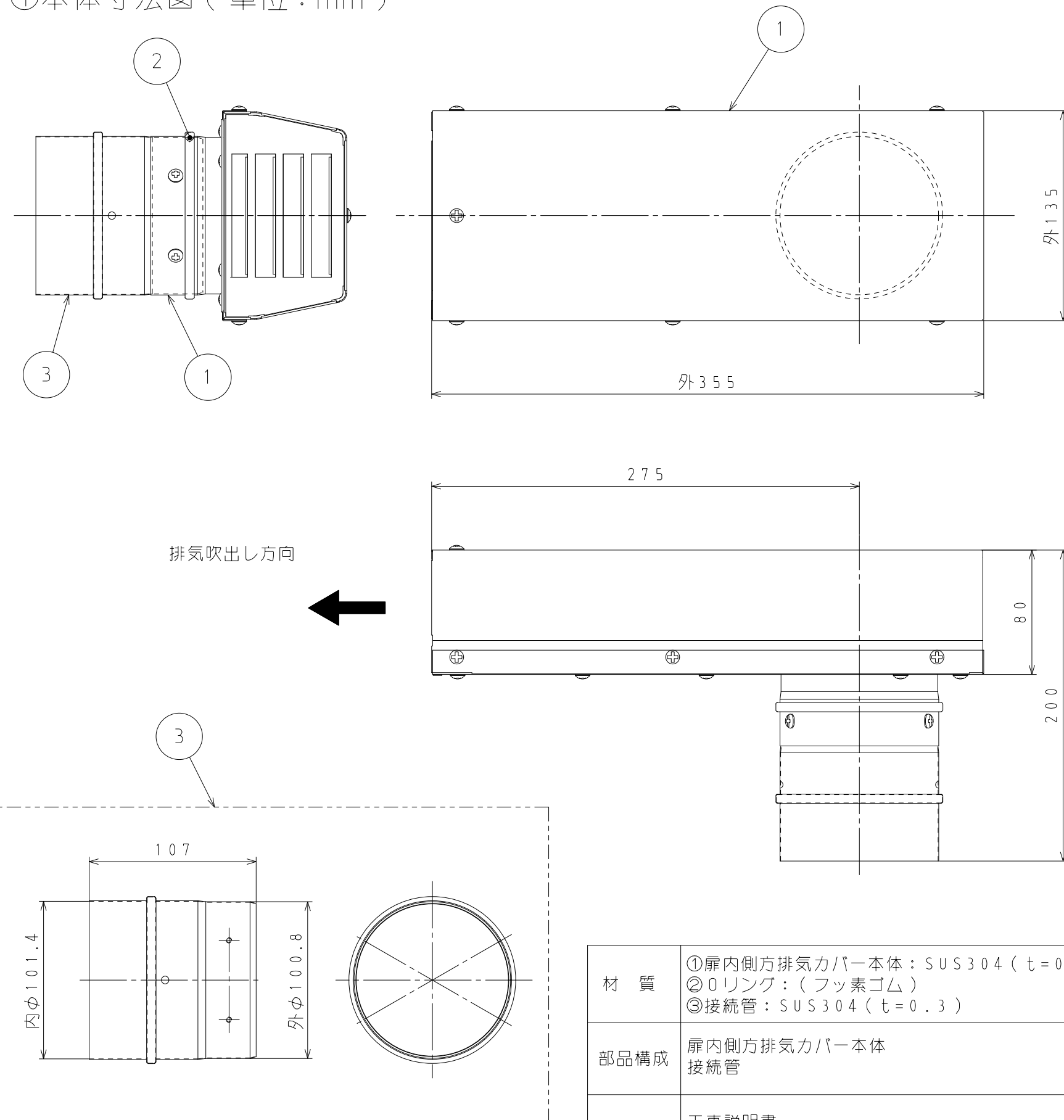
①本体寸法図（単位：mm）
