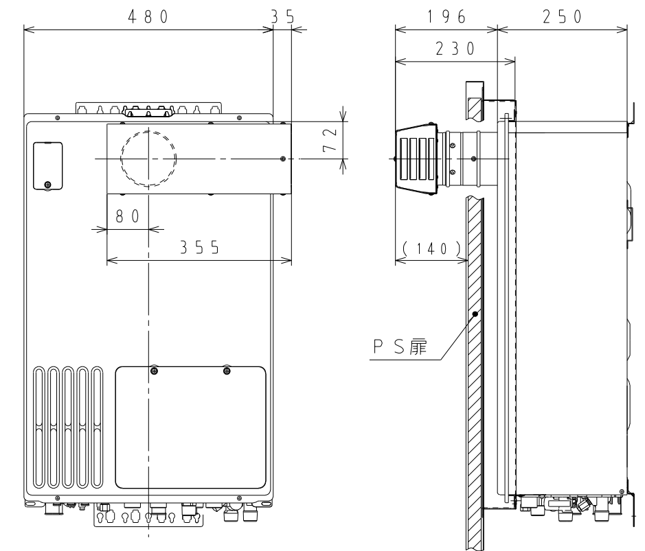
取付例（図は右吹出しを示す）
