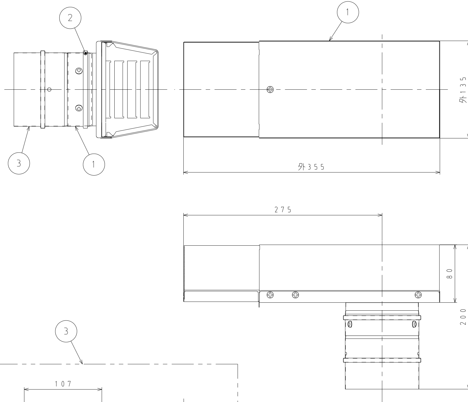
①本体寸法図（単位：mm）
