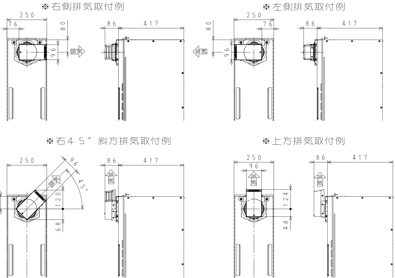
③GH-H241Z(A)WS 取付寸法図 (XT4219LRSシリーズ)
