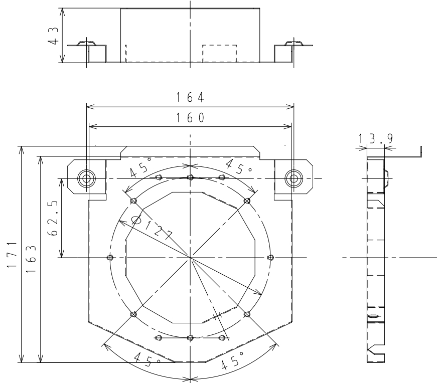
②取付金具寸法図（単位：mm）
