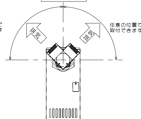
斜方排気取付
