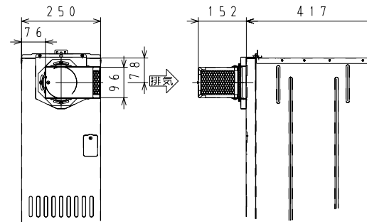
※右側排気取付例
