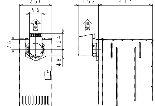
※上方排気取付例
