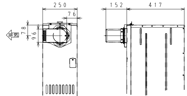
※左側排気取付例
