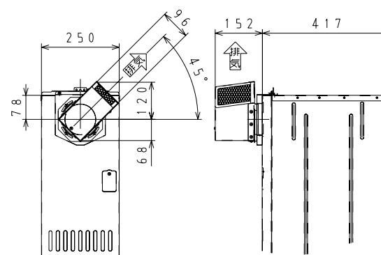
※右45°斜方排気取付例
