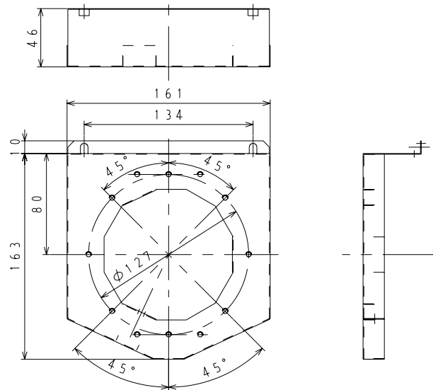
②取付金具寸法図 (単位: mm)
