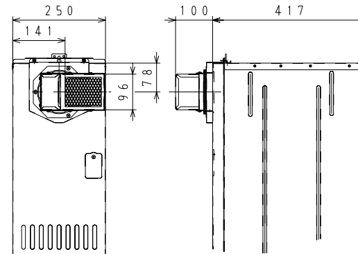
※右側排気取付例
