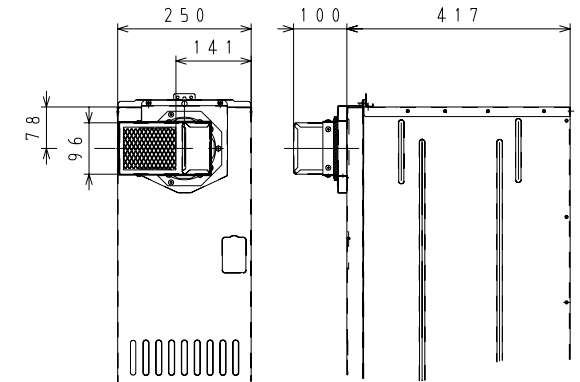
※左側排気取付例
