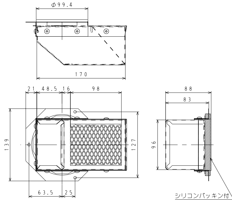
②取付金具寸法図 (単位: mm)
