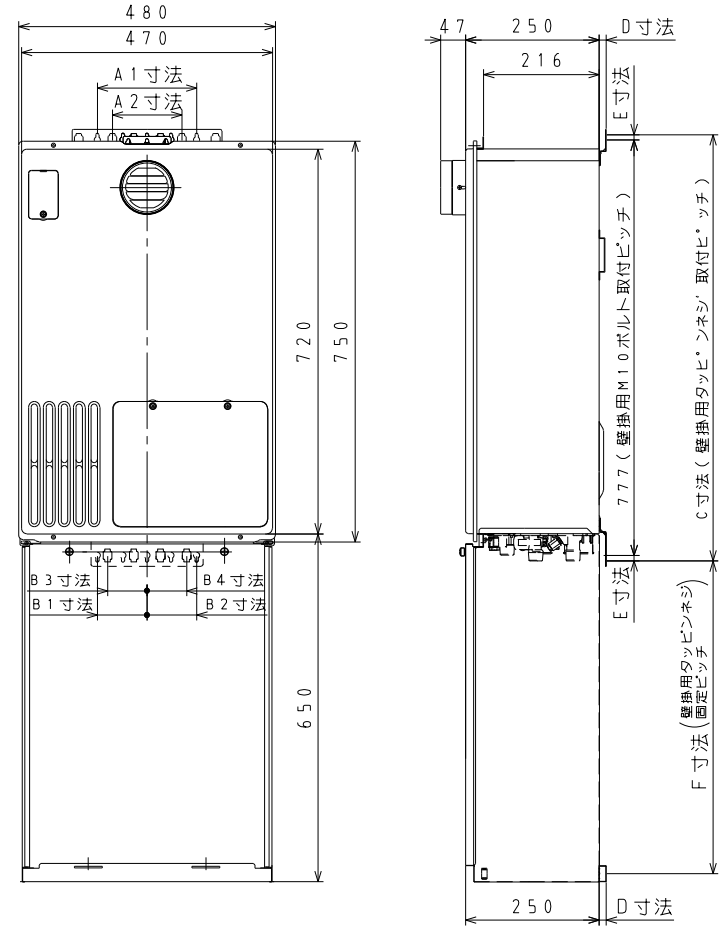
取付け寸法図
