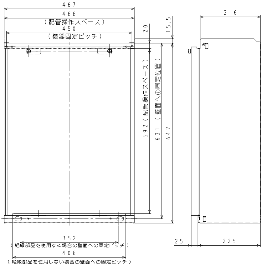
① 寸法図 (単位: mm)
