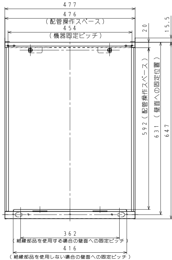
① 寸法図 (単位: mm)
