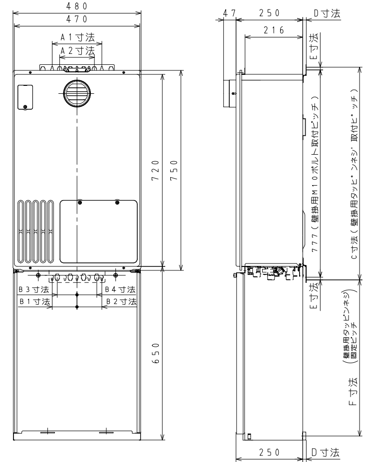
② XT4214ARSAW3CU 取付け寸法図
